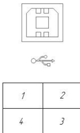
Рисунок 1.6 – Разъем USB тип В порта USB
