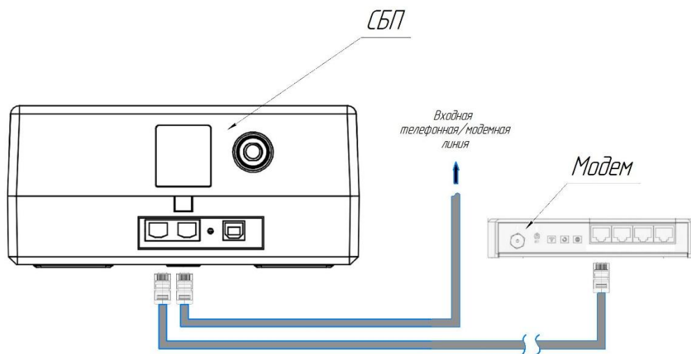
Рисунок 1.5 – Схема подключения телефонной или модемной линии к СБП
