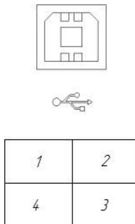
Рисунок 1.3 – Разъем USB тип В порта USB
