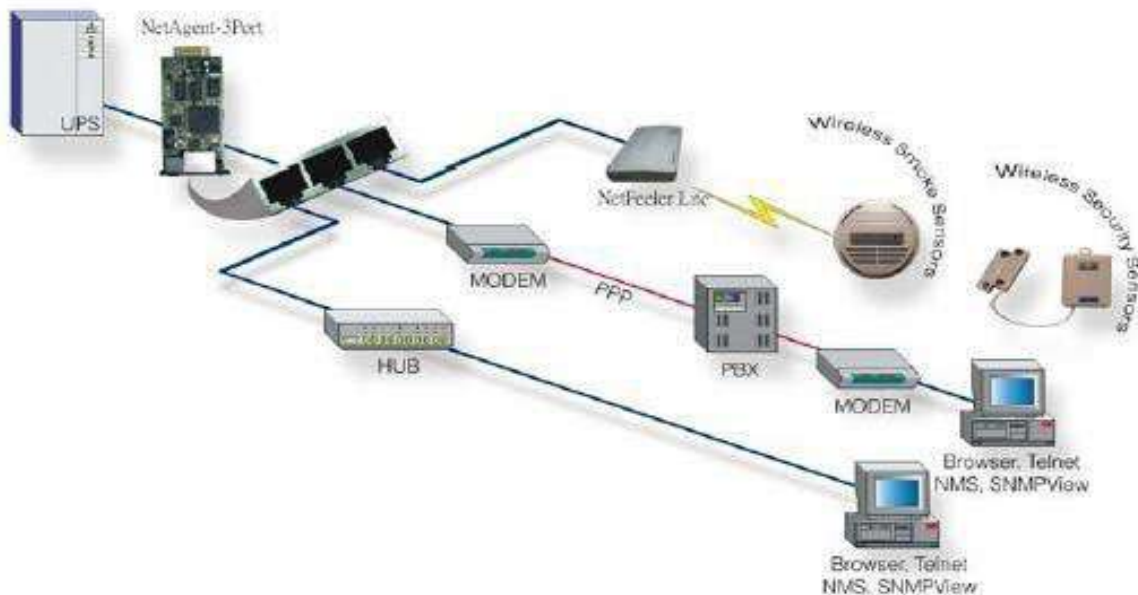
Топология сетевого управления СБП
